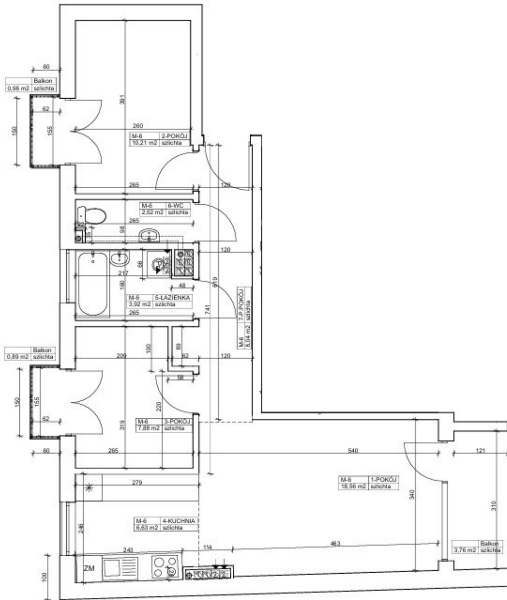
RZUT 2 PIĘTRA 1:500
