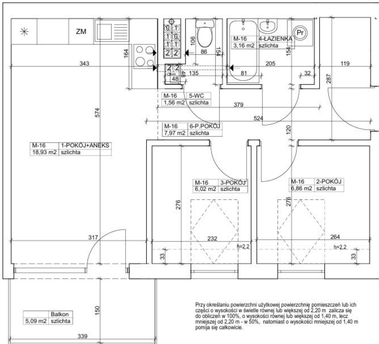
RZUT 2 PIĘTRA 1:500
