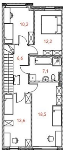
RZUT PIĘTRA
