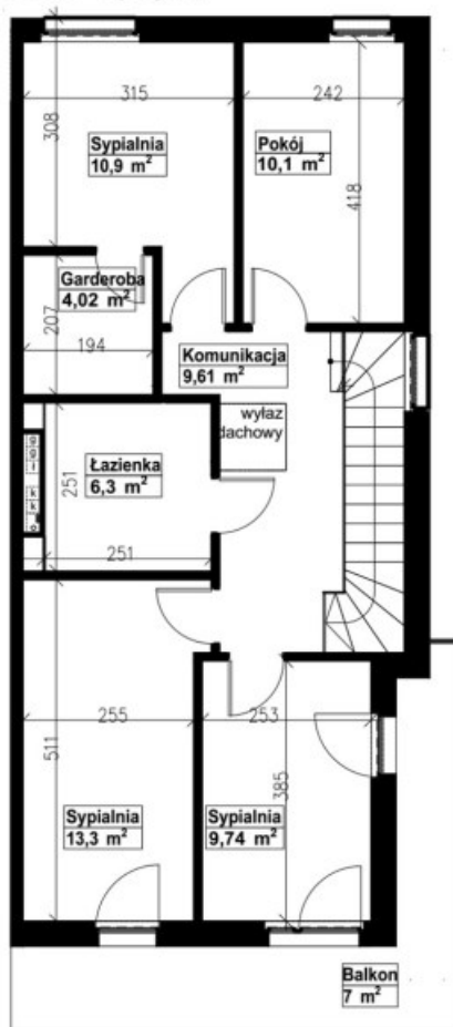
Rzut 1 piętra
