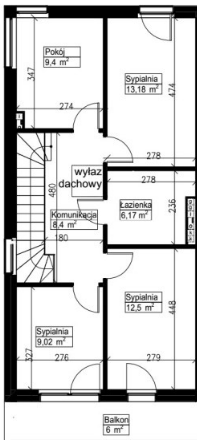
Rzut 1 piętra
